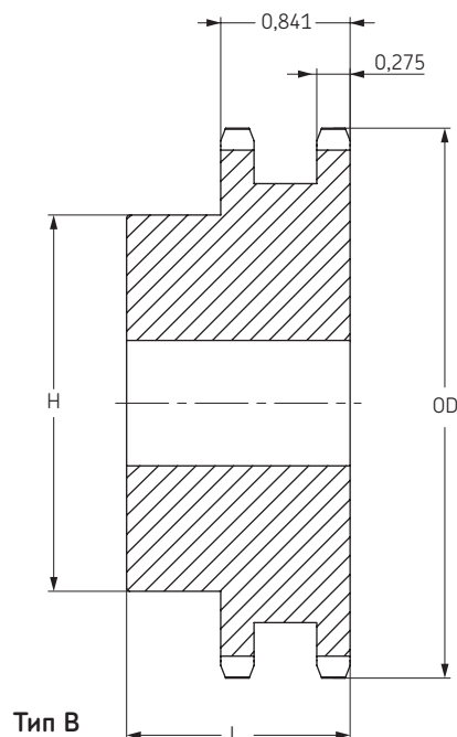
ANSI 40-2 Шаг 1/2"
