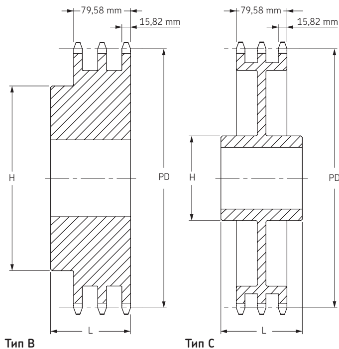
ISO 16B-3 Шаг 25,40 мм
