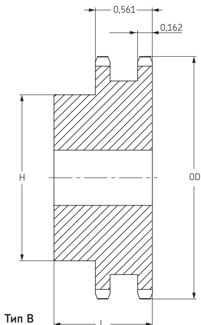
ANSI 35-2 Шаг 3/8"
